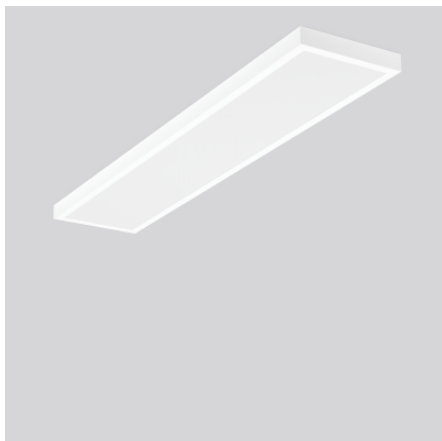
Deckenleuchten 4068754002714 L 1562, B 325, H 54
