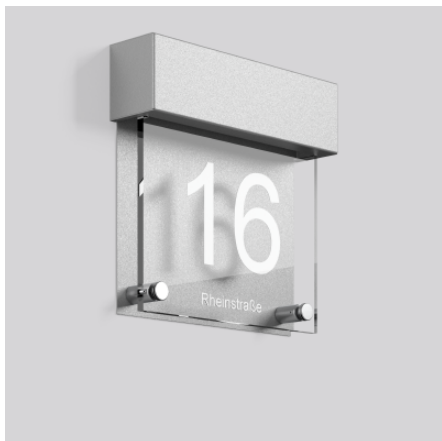
Hausnummernleuchten 4051859999140 L 250, B 48, H 255
