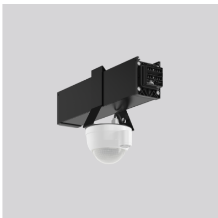
Lichtbandmodul 4051859963783 L 330, B 165, H 120
