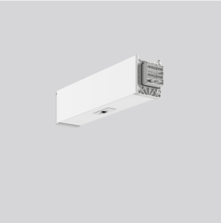
Lichtbandmodul 4051859657590 L 330, B 58, H 76 Leuchteinbau verkehrsweiß, matt (RAL 9016)
