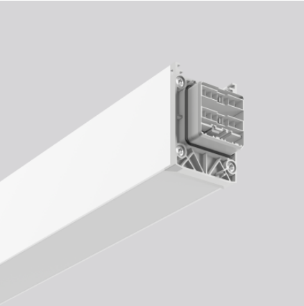
Lichtbandmodul 4051859626084 L 598, B 58, H 76 Deckenanbau, Ketten- oder Seilpendel verkehrsweiß, matt (RAL 9016)
