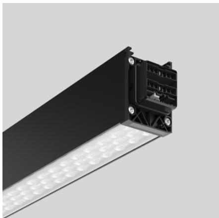
Lichtband 4051859638407 L 598, B 58, H 76
