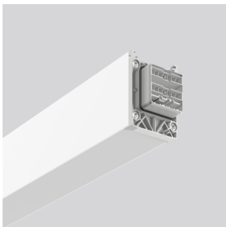
Lichtbandmodul 4051859941385 L 818, B 58, H 76
