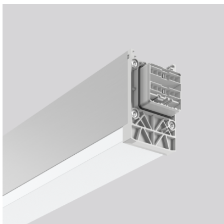
Lichtband 4051859555834 L 1163, B 58, H 91
