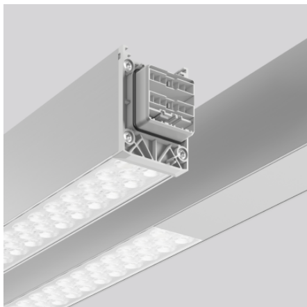
Lichtband 4051859629887 L 2291, B 58, H 76
