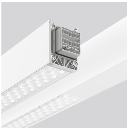
Lichtband 4051859629740 L 2291, B 58, H 76
