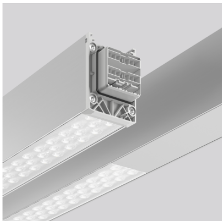
Lichtband 4051859567721 L 4547, B 58, H 76
