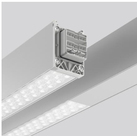
Lichtband 4051859570042 L 4547, B 58, H 76
