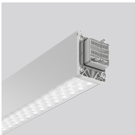
Lichtband 4051859506416 L 4547, B 58, H 76
