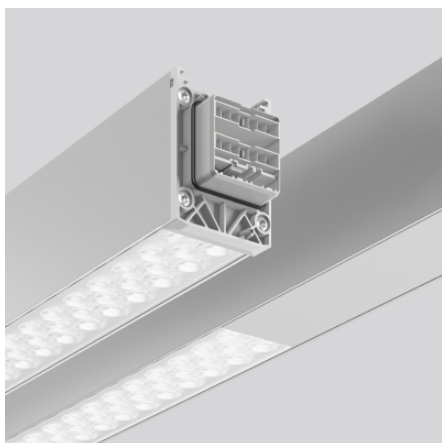
Lichtband 4051859604891 L 4547, B 58, H 76
