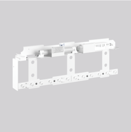
LED Umrüstsatz 4051859983279 L 430, B 60, H 140
